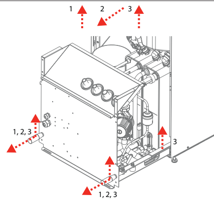
4. Dra ut kylmodulen genom att med hjälp av bärhandtagen först lyfta modulen något uppåt.
