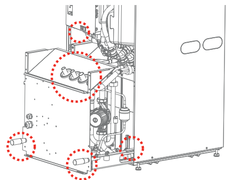
6. Lyft in kylmodulen i produkten med hjälp av bärhandtag och bärremmar. Lossa bärhandtag samt återmontera elkabelkontakt, slangar och skruvar.
