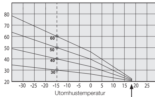
Framledningstemperatur
