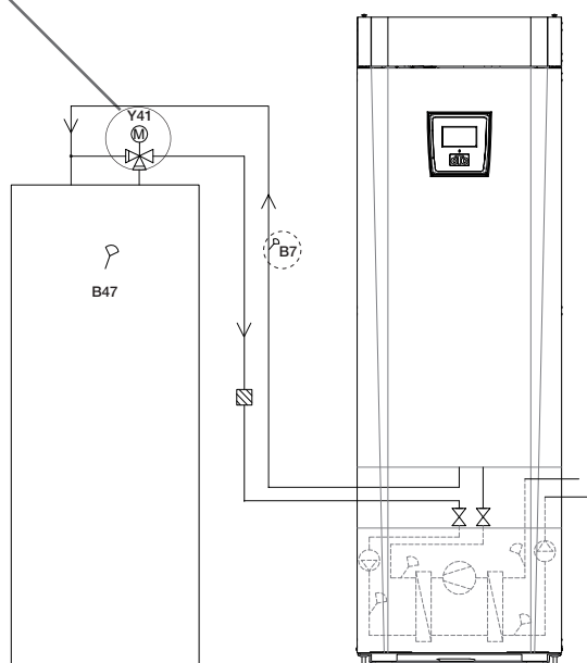
Shuntventil trevägs VRG 131
