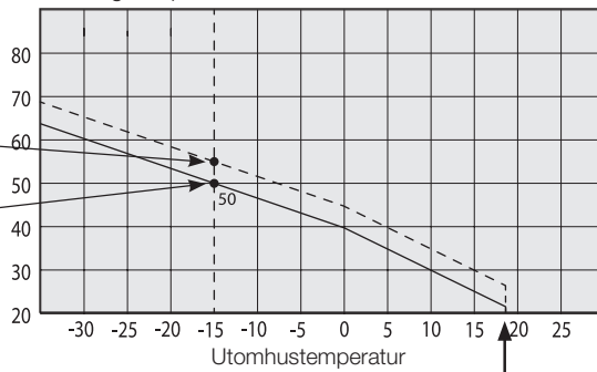
Framledningstemperatur
